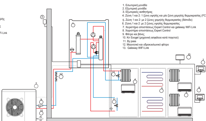
ARIANEXT PLUS M 2Ζώνες
