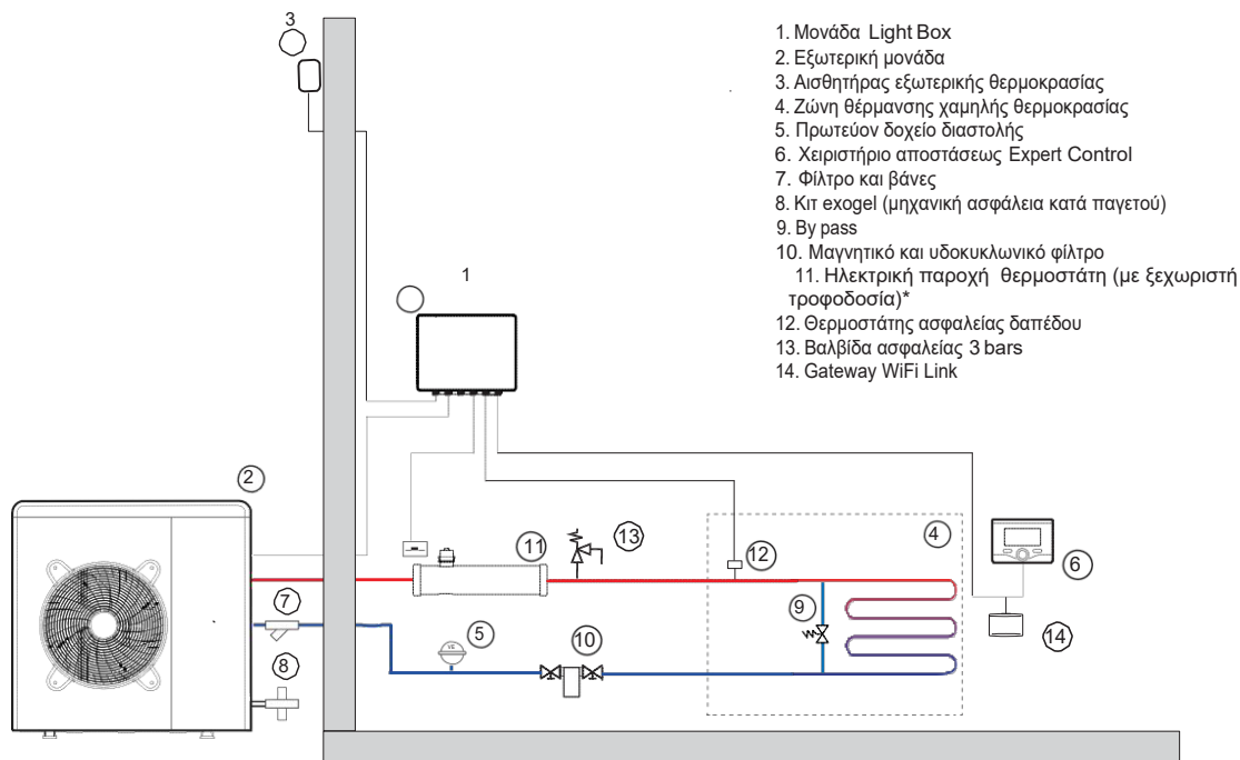
ΥΔΡΑΥΛΙΚΟ ΣΧΗΜΑ ARIANEXT LITE M – Θέρμανση δαπέδου
