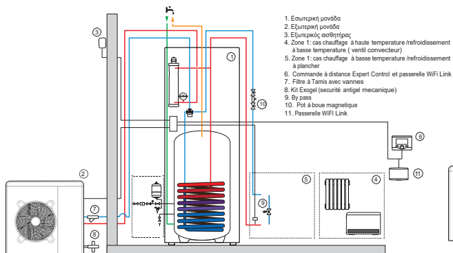
ARIANEXT COMPACT M 1Ζώνη
