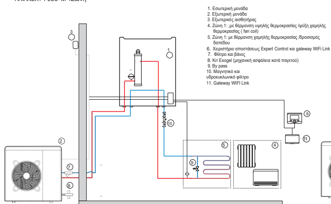
ARIANEXT PLUS M 1Ζώνη
