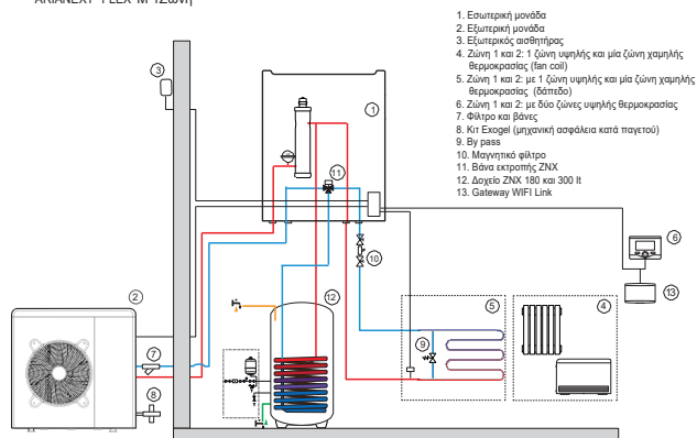
ARIANEXT FLEX M 1Ζώνη
