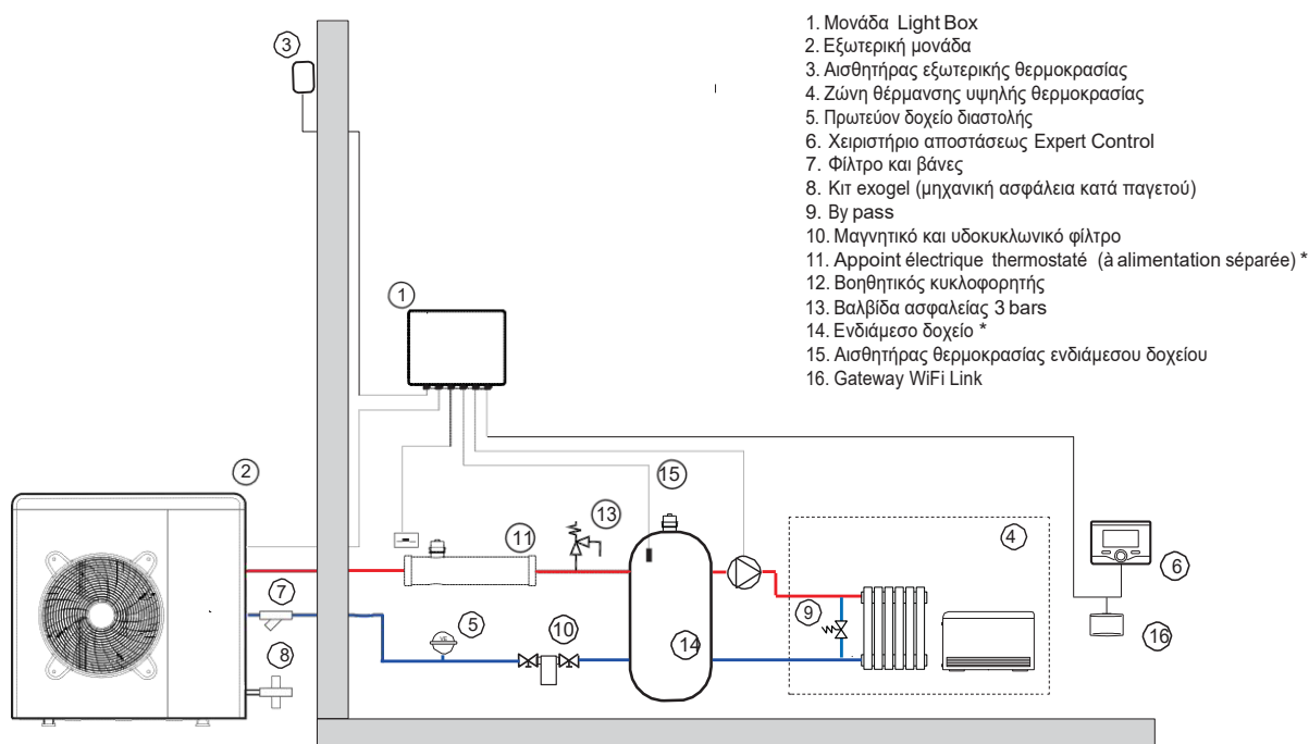
ΥΔΡΑΥΛΙΚΟ ΣΧΗΜΑ ARIANEXT LITE M – Σώματα με ενδιάμεσο δοχείο
