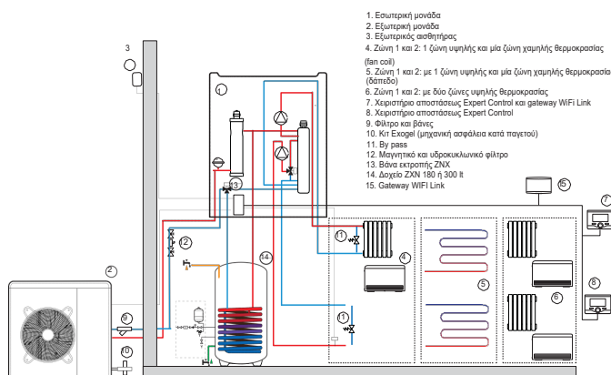
ARIANEXT FLEX M 2Ζώνες
