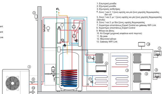
ARIANEXT COMPACT M 2Ζώνες
